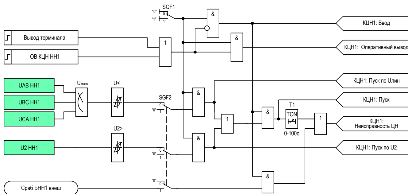
Рисунок 2.11 – Функциональная схема логики КЦН НН1
