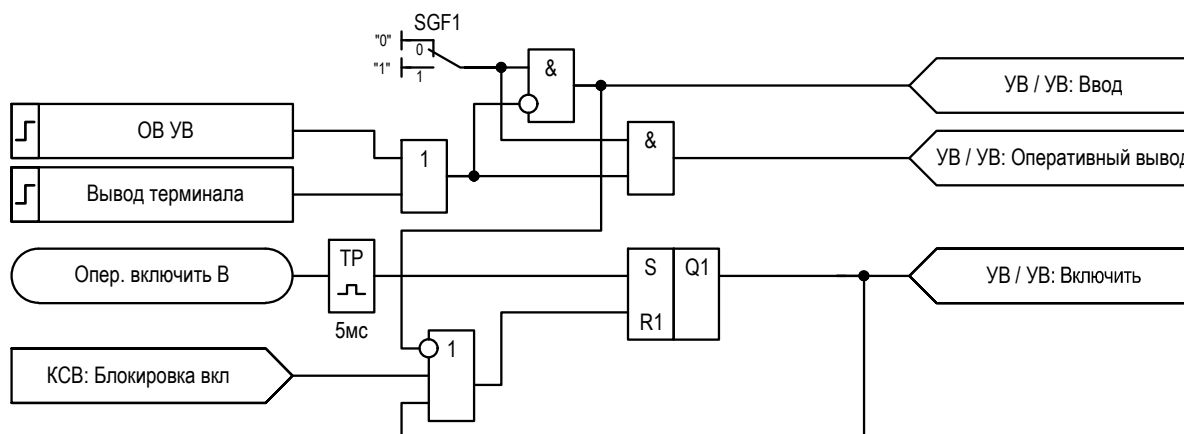
Рисунок 2.25 – Функциональная схема логики УВ
