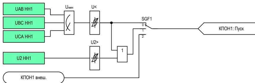
Рисунок 2.2 – Функциональная схема логики КПОН1
