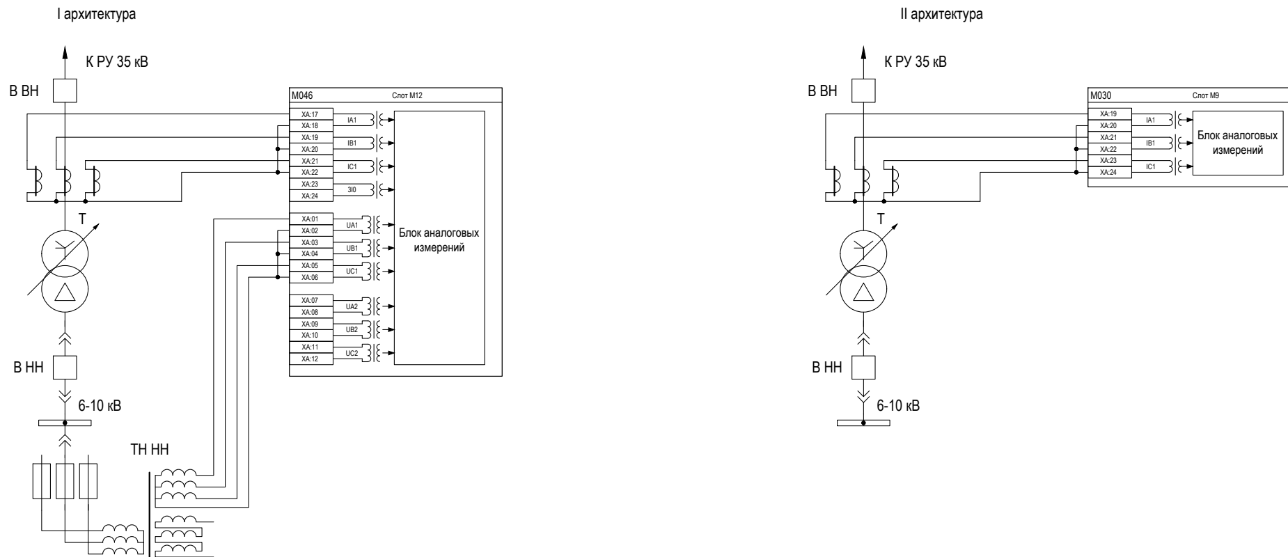
Рисунок Г.1 – Подключение аналоговых цепей трансформаторов тока и напряжения двухобмоточного трансформатора 35 кВ к устройству
