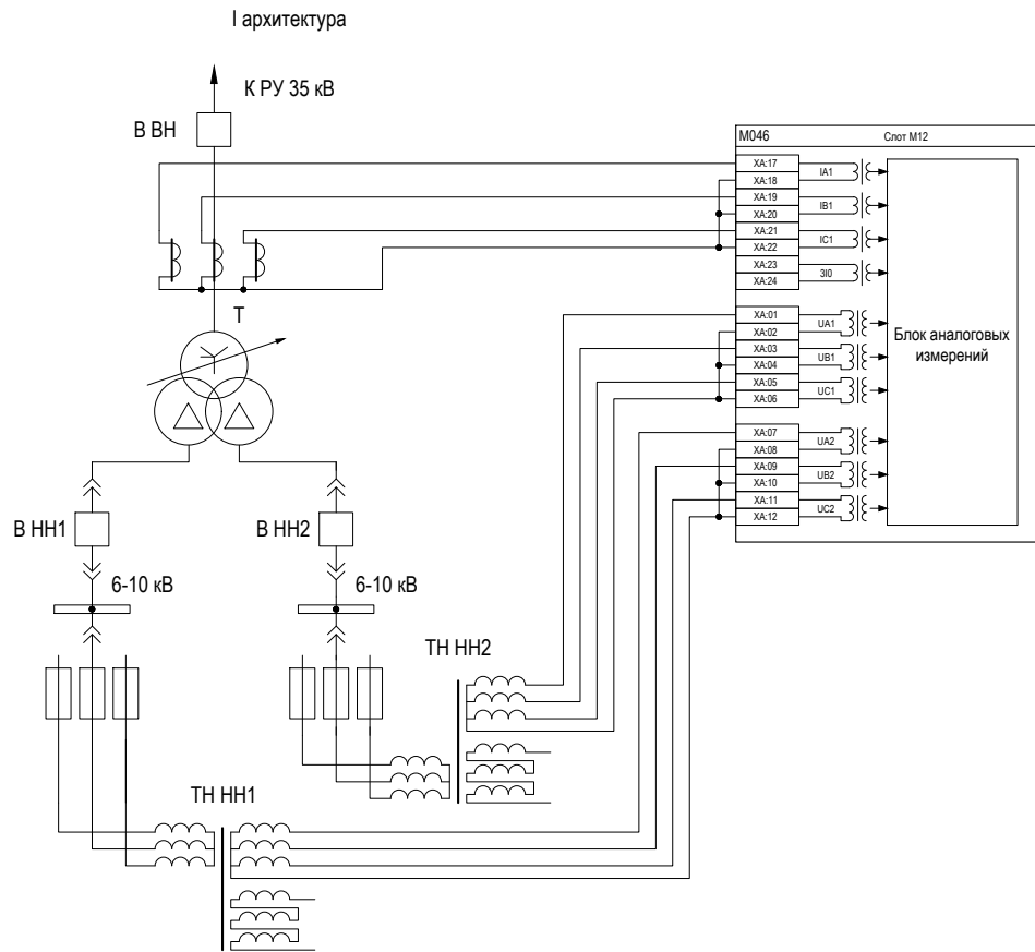
Рисунок Г.2 – Подключение аналоговых цепей трансформаторов тока и напряжения трансформатора 35 кВ с расщепленной обмоткой низшего напряжения к устройству
