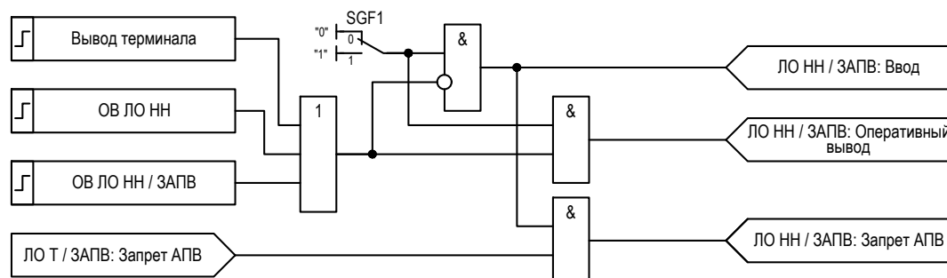
Рисунок 2.18 – Функциональная схема логики запрета АПВ
