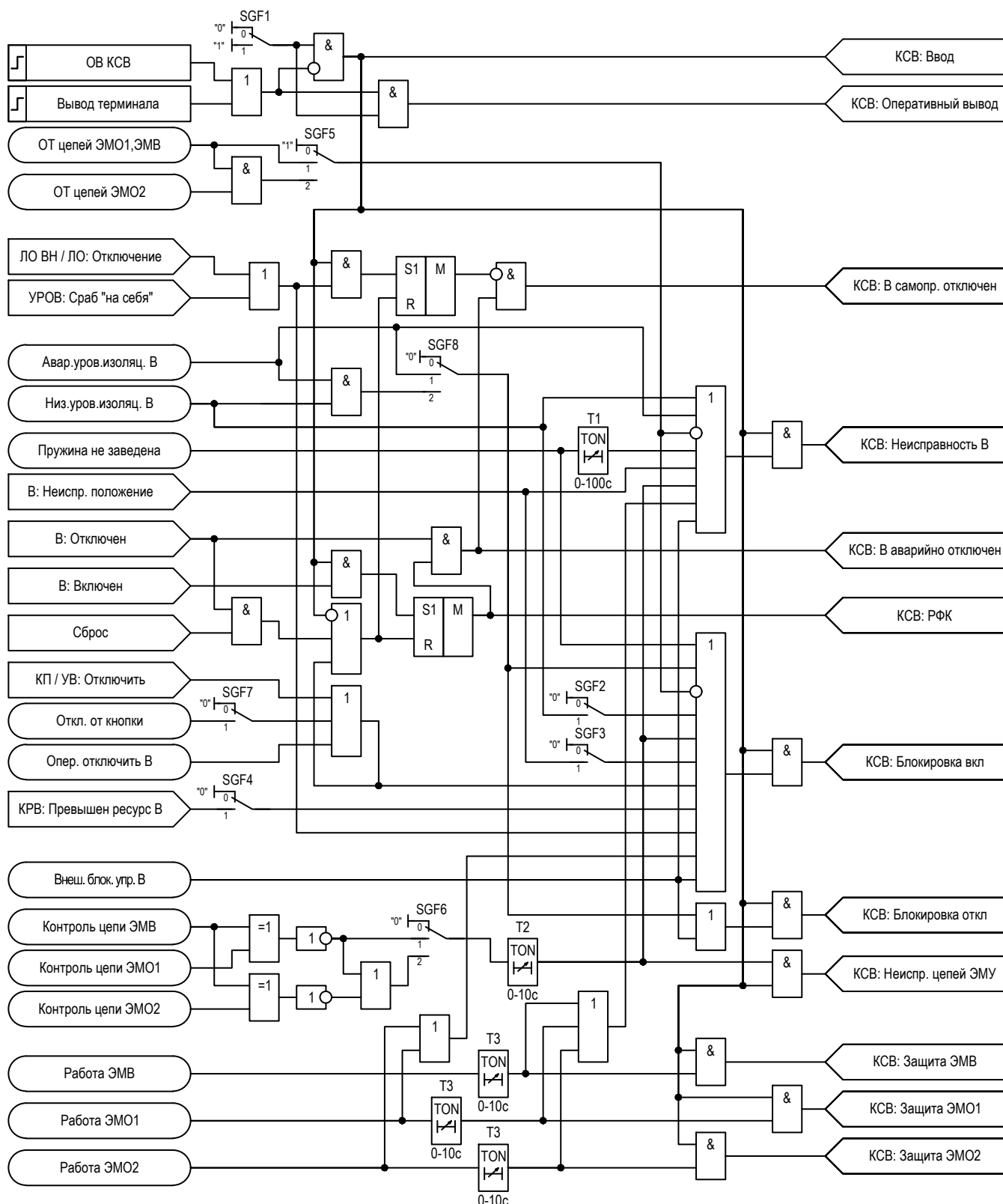
Рисунок 2.22 – Функциональная схема логики КСВ
