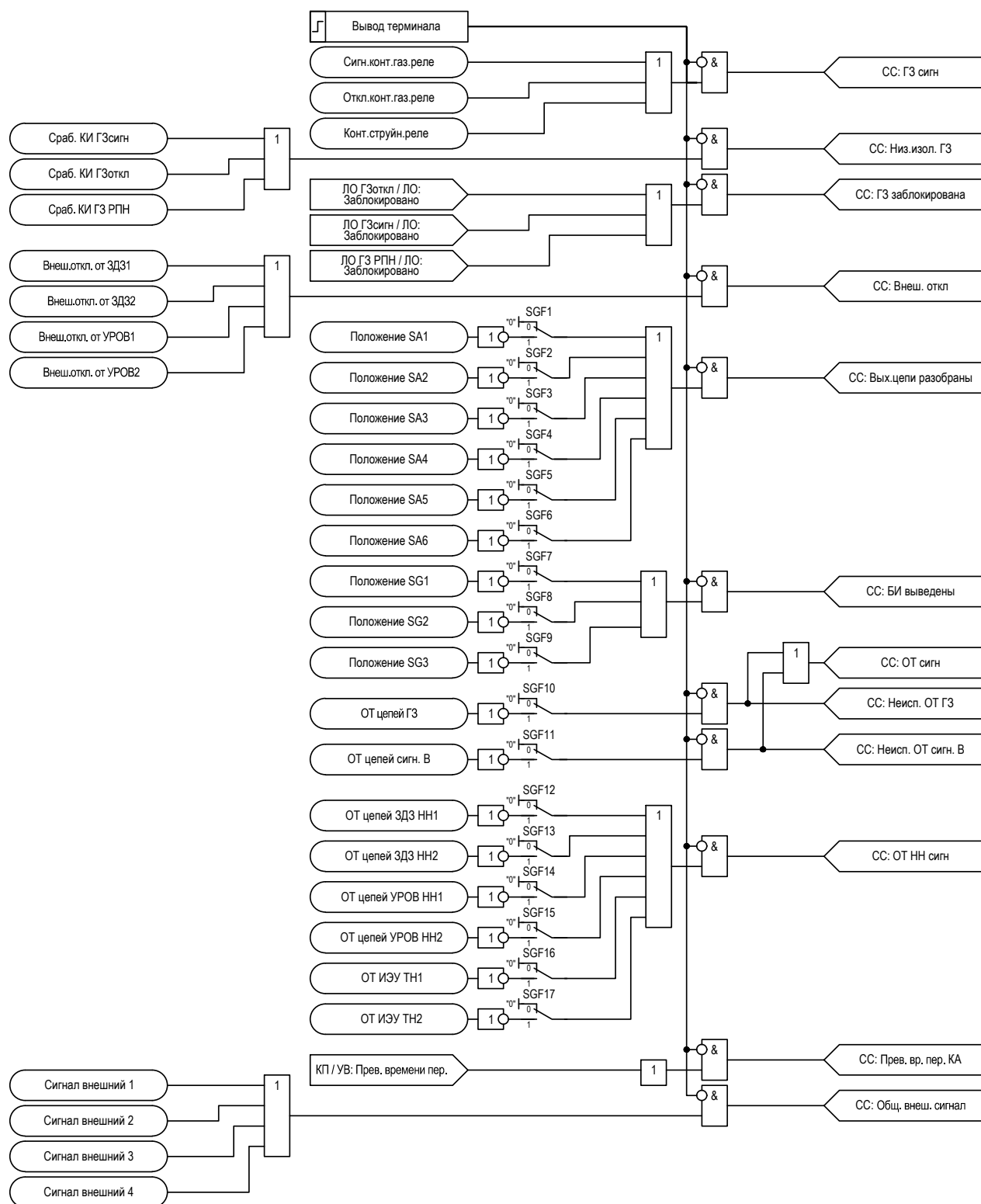
Рисунок 2.28 – Функциональная схема логики сборки сигналов
