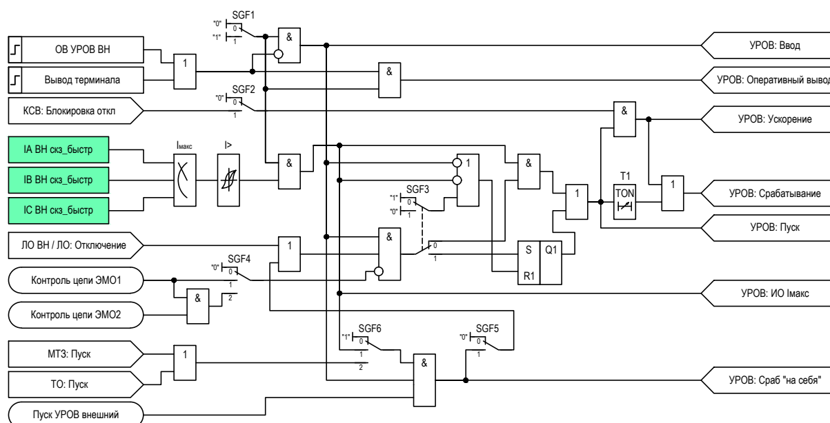
Рисунок 2.20 – Функциональная схема логики УРОВ
