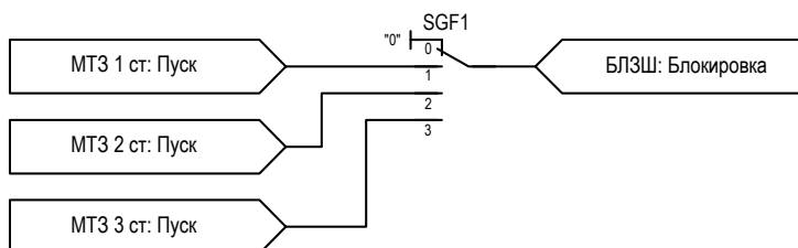
Рисунок 2.4 – Функциональная схема логики БЛЗШ
