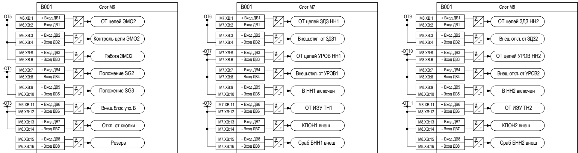
Рисунок Д.3 – Подключение дискретных входов и выходов к внутренним сигналам алгоритмов для блоков в слотах М6-М8
