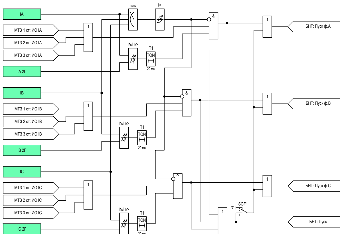
Рисунок 2.3 – Функциональная схема логики БНТ
